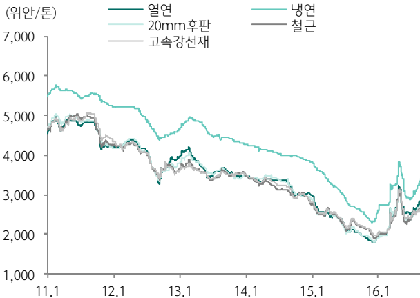
그림 5. 중국 철강 유통가격 추이
