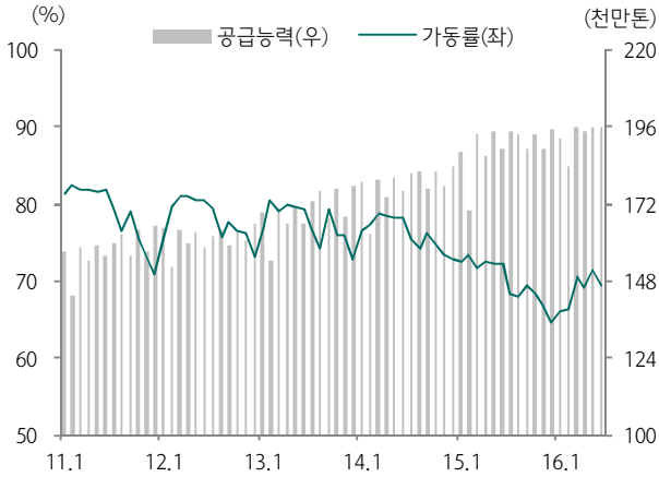
그림 1. 전세계 철강 가동률 추이
